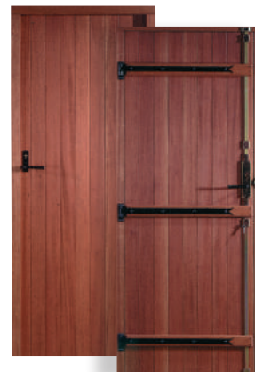
Modèle exotique, frises verticales pas de 27 mm , option serrure de sûreté à cylindre 3 points, ouverture intérieure .
