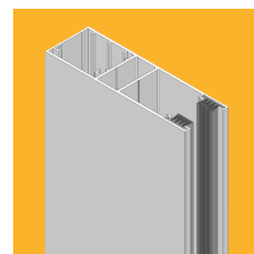
Coulisse en aluminium avec joints brosse
