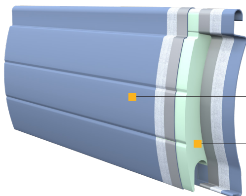
Lame aluminium profilé double paroi
